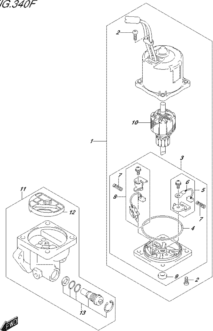
FIG.340F (2-F-8) PTT MOTOR (DF140AT E11)
